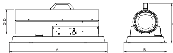
GRY – D H Generador de aire caliente con asa por combustión directa.
